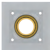
Płyta S wymiary: 54x54 cm
